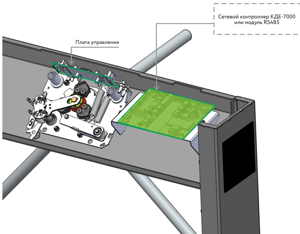
Рисунок 2.5 – Расположение элементов системы в корпусе турникета 3V
